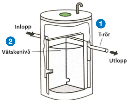
Tvärsnitt av en trekammarbrunn.
